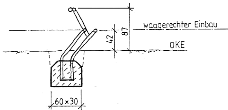
SEITENANSICHT
