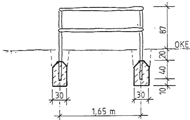
VORDERANSICHT
